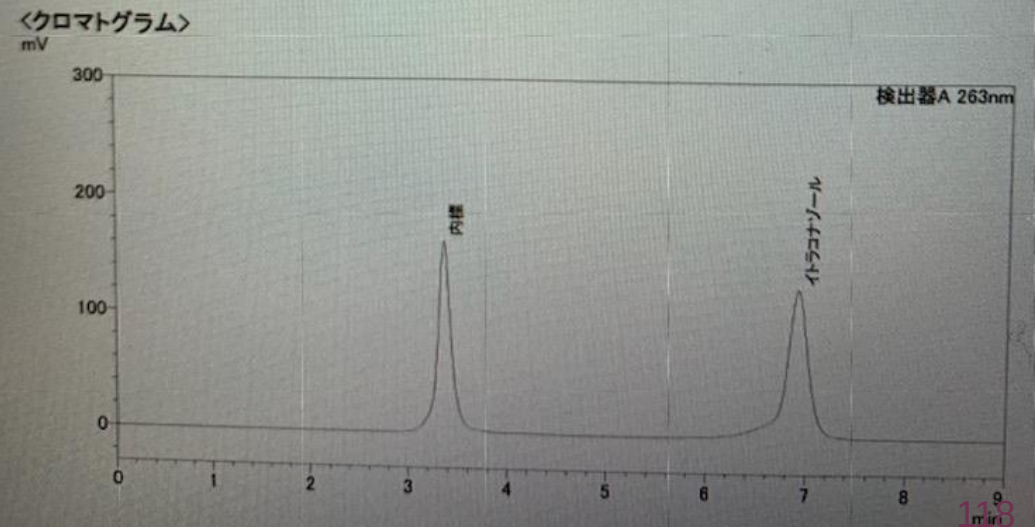
【標準溶液の液体クロマトグラム】
